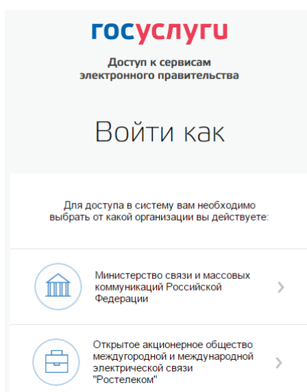
Рисунок 37 – Выбор роли
